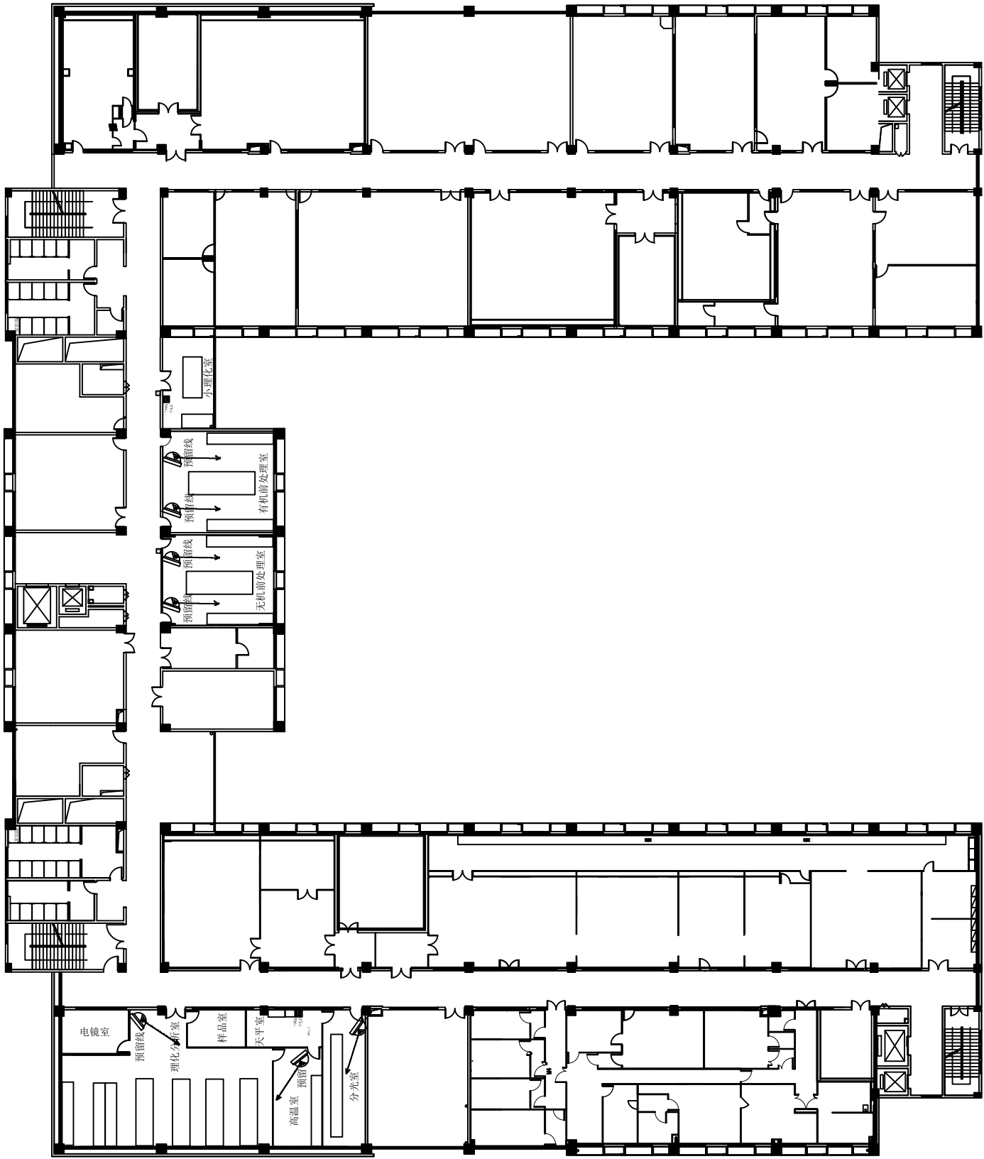
纤检楼二楼平面图
